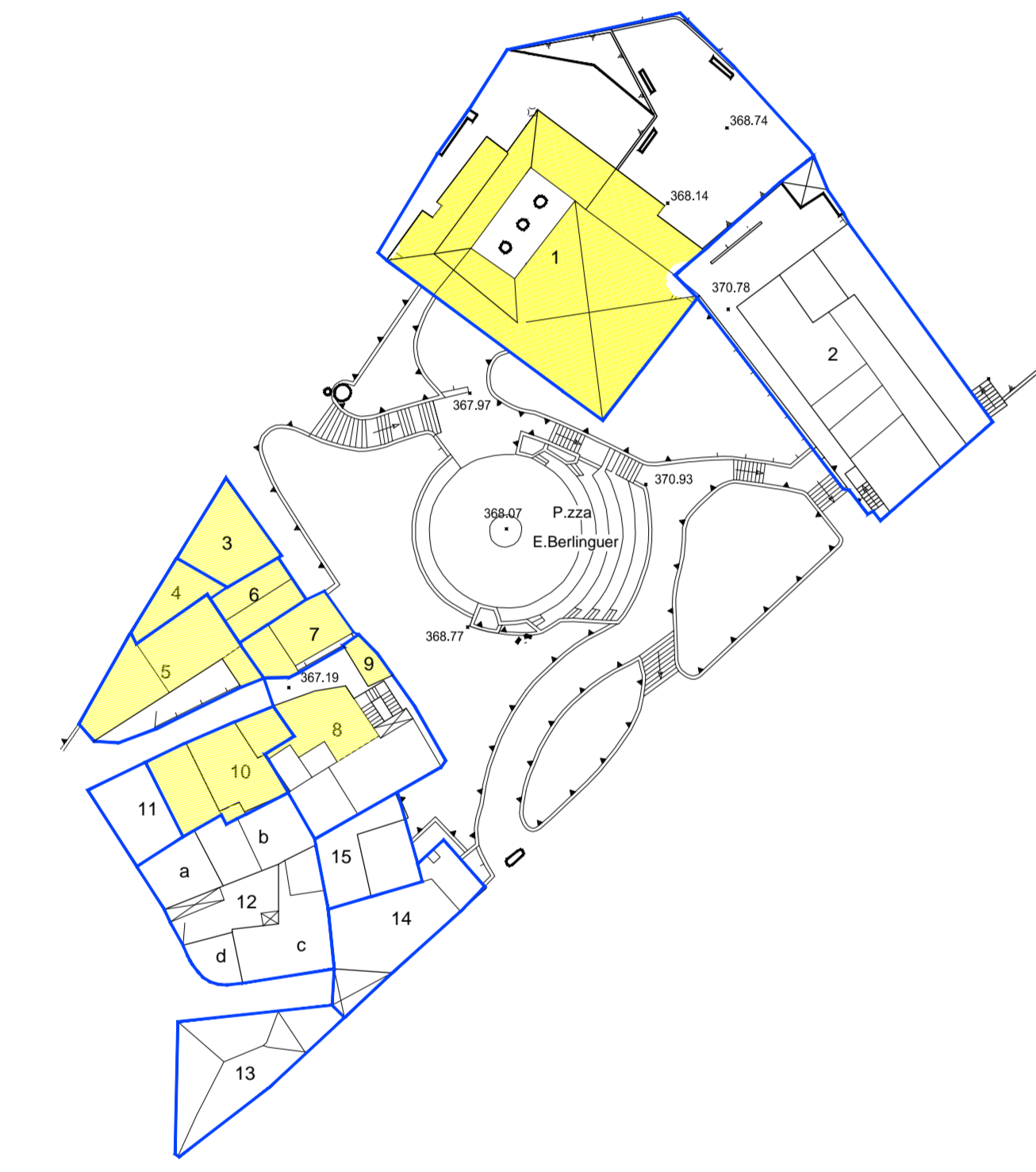
PLANIMETRIA PRIMO LIVELLO
